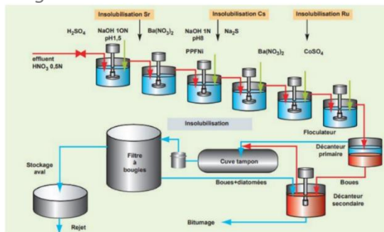
Diagramme du procédé de traitement des effluents de STE3 La Hague
