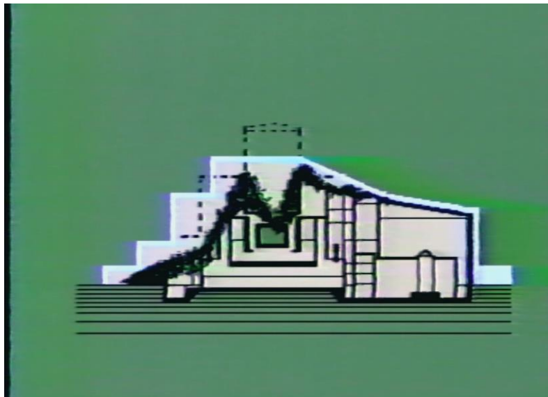
Figure 5 : Enceinte de confinement, extrait du film Tchernobyl du Comité d'Etat de l'Union soviétique pour l'utilisation de l'énergie atomique, 1986. Archives IRSN/FAR 380318.
