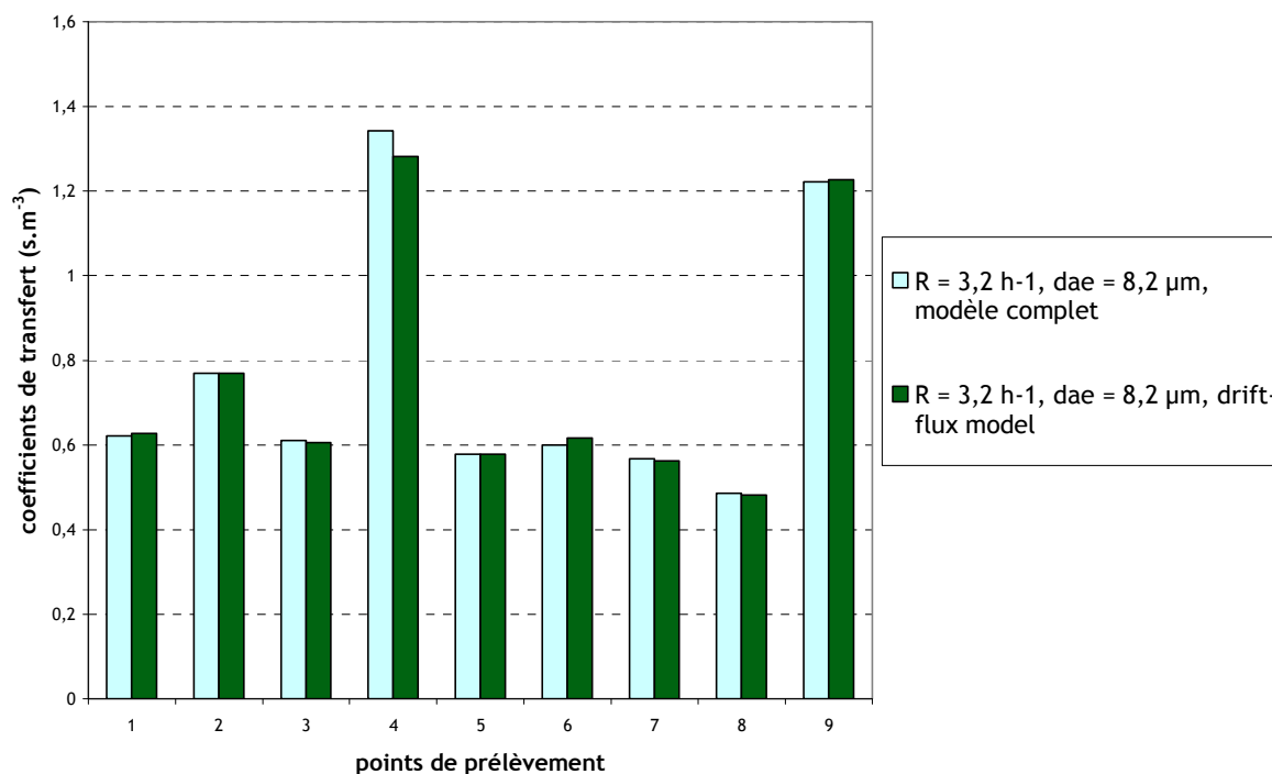
figure 165. Coefficients de transfert de particules obtenus par simulations dans le local expérimental de 1575 m 3 . R = 3,2 \text{ h}^{-1} , d_{ae} = 8,2 \text{ }\mu\text{m} . Influence du modèle de transport de concentration
