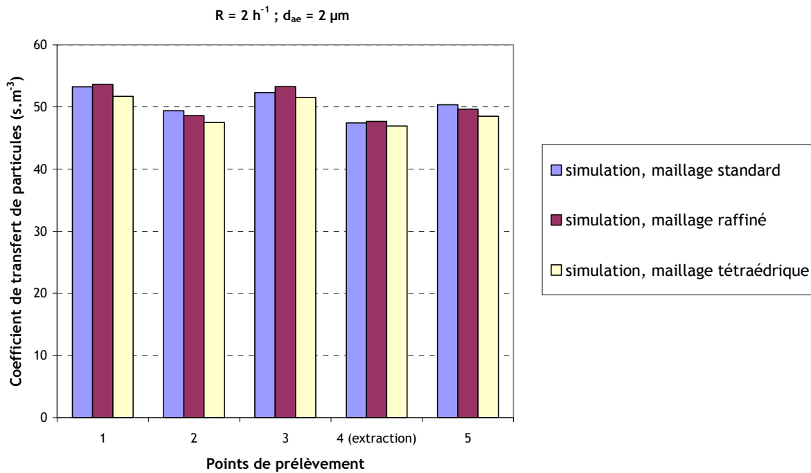
figure 136. Résultats de simulations effectuées dans le local CEPIA. Maillage standard, R = 2 \text{ h}^{-1} , d_{ae} = 2 \text{ }\mu\text{m} . Influence du maillage utilisé
