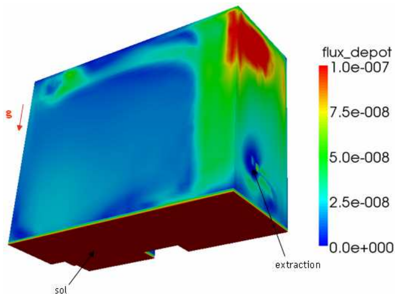
figure 143. Flux surfacique de dépôt obtenu par simulation dans le local CEPIA. Maillage standard, turbulence k-\epsilon avec D_H \text{ soufflage} = 0,12 \text{ m} , D_H \text{ injection} = 0,04 \text{ m} et I = 5 \% comme conditions limites aux entrées. Concentration à l'injection : 10 \text{ mg.m}^{-3} . Borne supérieure de l'échelle bloquée à 10^{-7} \text{ kg.m}^{-2}.\text{s}^{-1}
