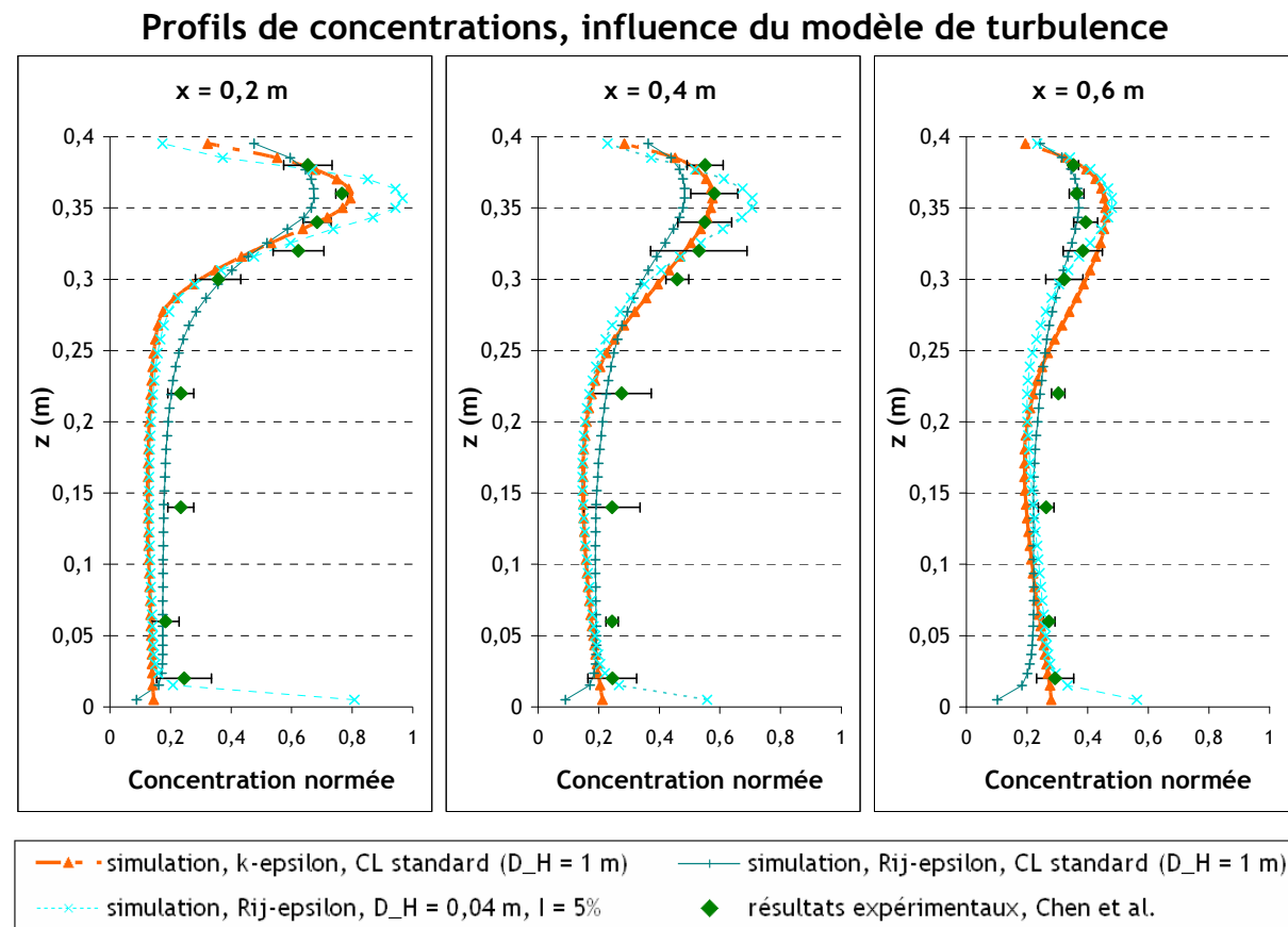
figure 85. Profils de concentrations normées ( C/C_0 ) obtenus pour U_x = 0,225 m.s -1 au soufflage (configuration 1), à trois distances x différentes de l'entrée. Influence du modèle de turbulence
