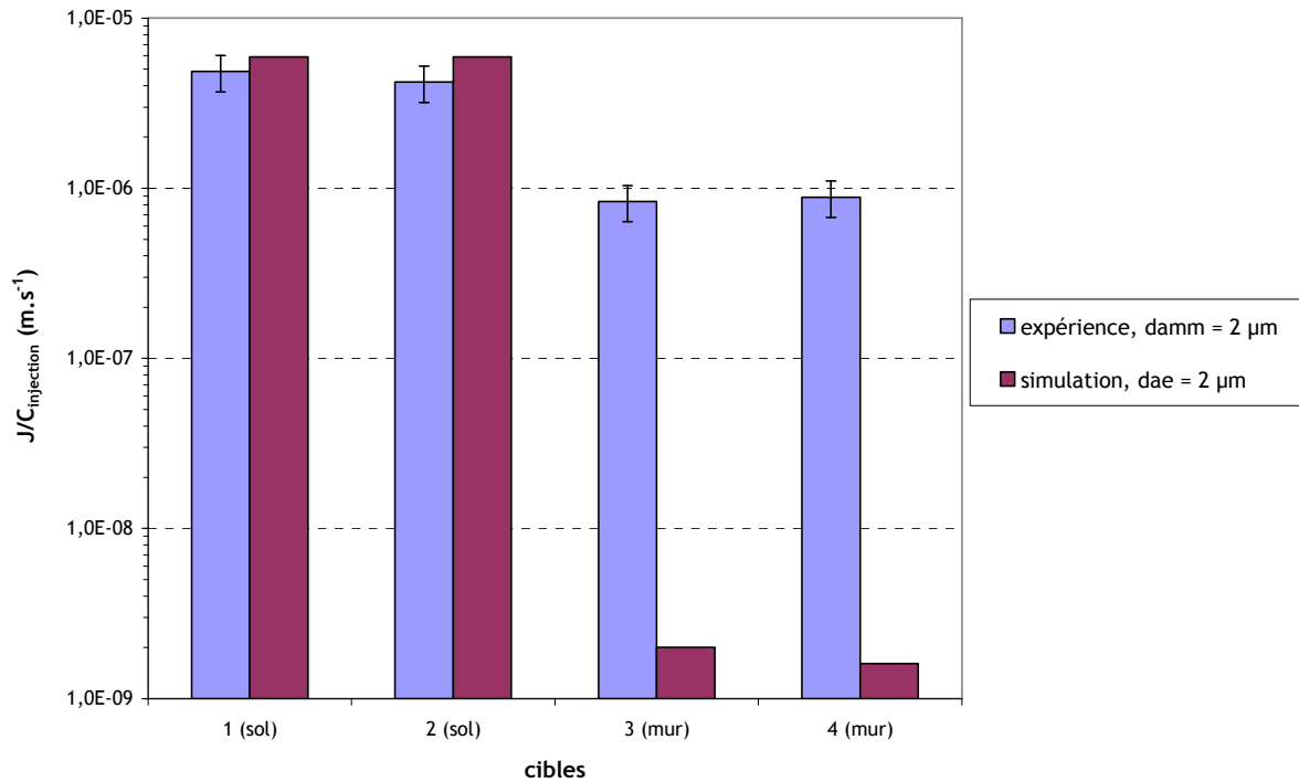
figure 142. Comparaison des flux de dépôt mesurés et calculés au sol dans le local CEPIA. Maillage standard, turbulence k-\epsilon avec D_H \text{ soufflage} = 0,12 \text{ m} , D_H \text{ injection} = 0,04 \text{ m} et I = 5 \% comme conditions limites aux entrées
