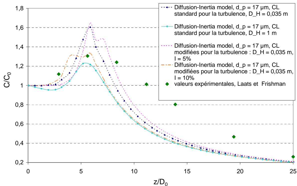
figure 75. Profil axial de concentration en aérosols de 17 \mu\text{m} dans un jet turbulent, normée par la concentration à l'injection C_0 . Modèle de turbulence k-\epsilon avec différentes conditions limites à l'injection
