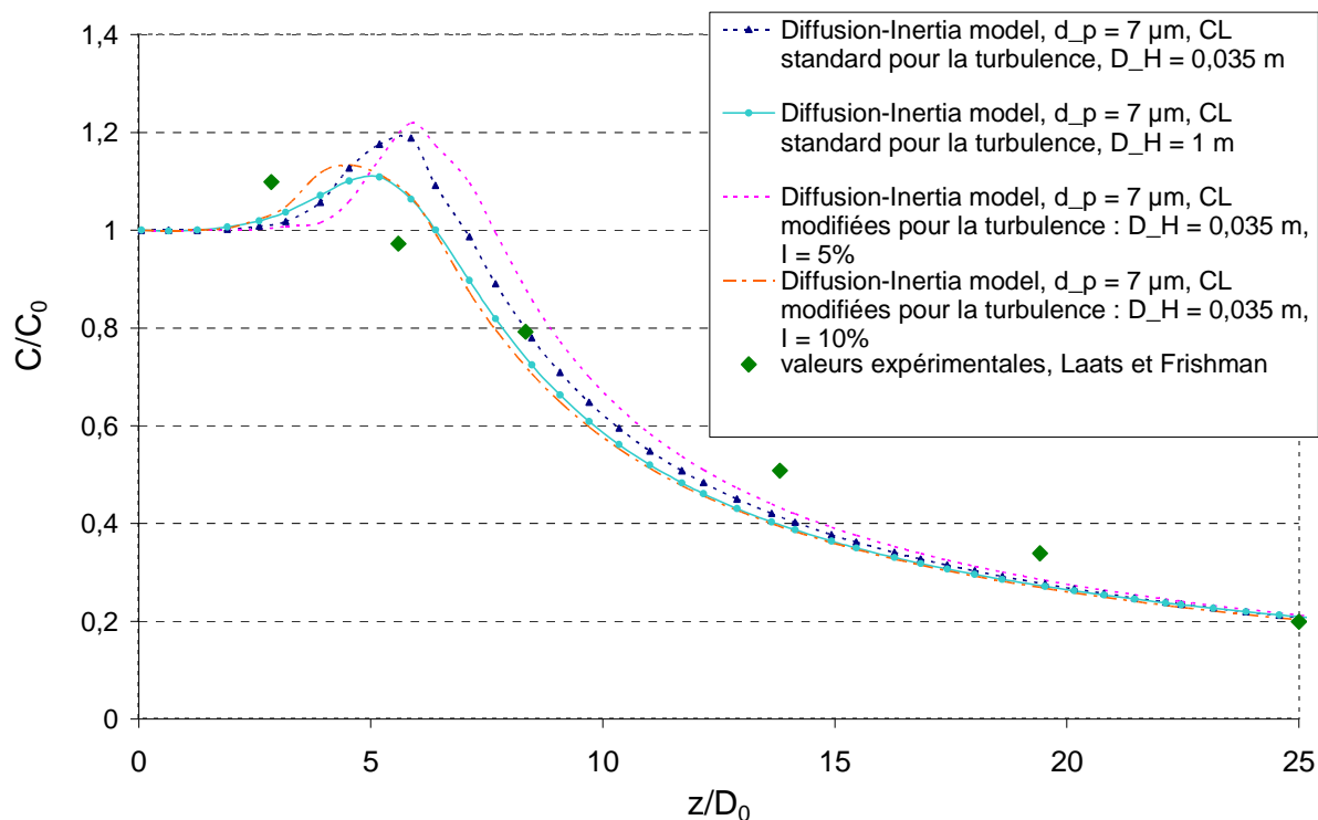
figure 74. Profil axial de concentration en aérosols de 7 \mu\text{m} dans un jet turbulent, normée par la concentration à l'injection C_0 . Modèle de turbulence k-\epsilon différentes conditions limites à l'injection
