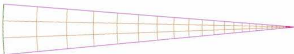
figure 174. Vue de la face d'entrée du maillage utilisé pour simuler la dispersion d'aérosols à la sortie d'un jet turbulent
