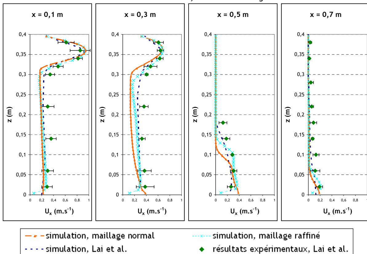
figure 97. Profils de concentrations normées ( C/C_0 ) obtenus pour U_x = 0,225 \text{ m.s}^{-1} au soufflage, à quatre distances x différentes de l'entrée. Influence du maillage utilisé
