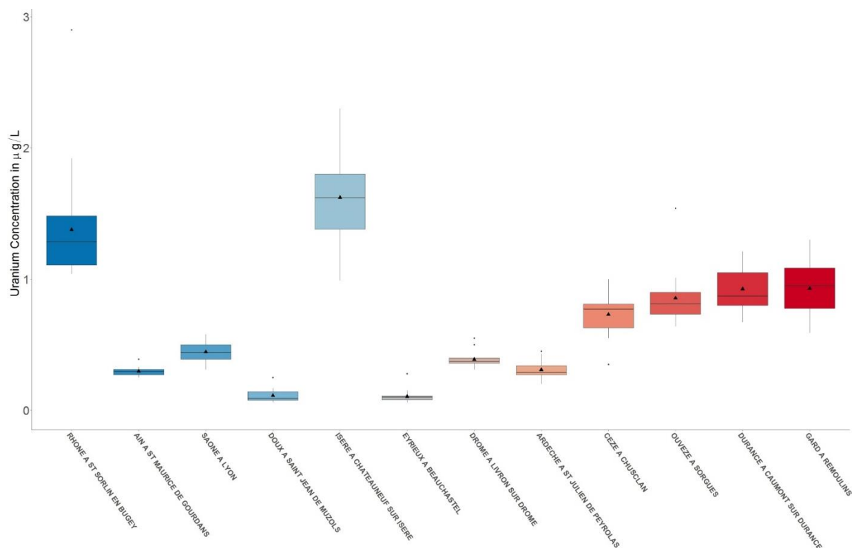
Figure III-11 : Boxplot concentrations en uranium naturel des principaux affluents du Rhône (configuration « Cast1.0 »). Données issues de http://www.naiades.eafrance.fr/ sur la période 2000-2020.
