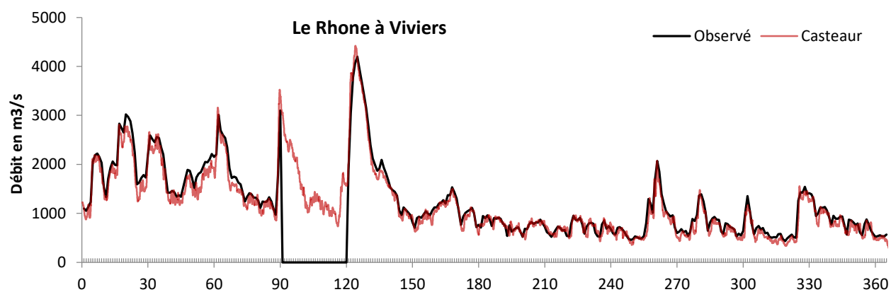
Figure III-3 : Comparaisons entre les débits simulés par Casteur et les débits observés (journaliers). De haut en bas : Stations de Perrache, Ternay, Valence, Viviers
