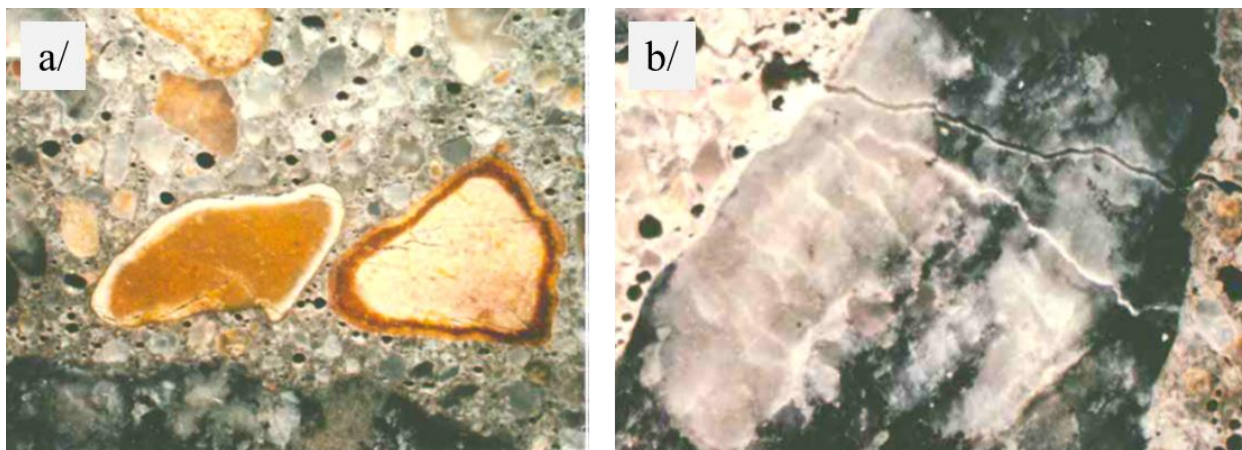
Figure 2 : a/ Auréole foncée de RAG autour d'un petit granulat de gneiss de granite (côté droit de l'image) inclus la matrice cimentaire[16]. b/ Fissure de RAG dans un granulat de gneiss de granite. En dessous la fissure principale, des fissures remplies de gel (en blanc) sont visibles[16].
