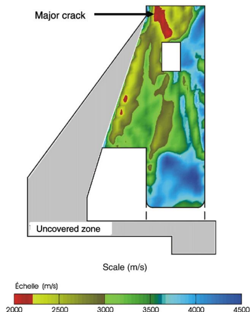
Figure 14 : Cartographie des vitesses ultrasonores (ondes longitudinales) sur un barrage atteint par la RAG [53].
