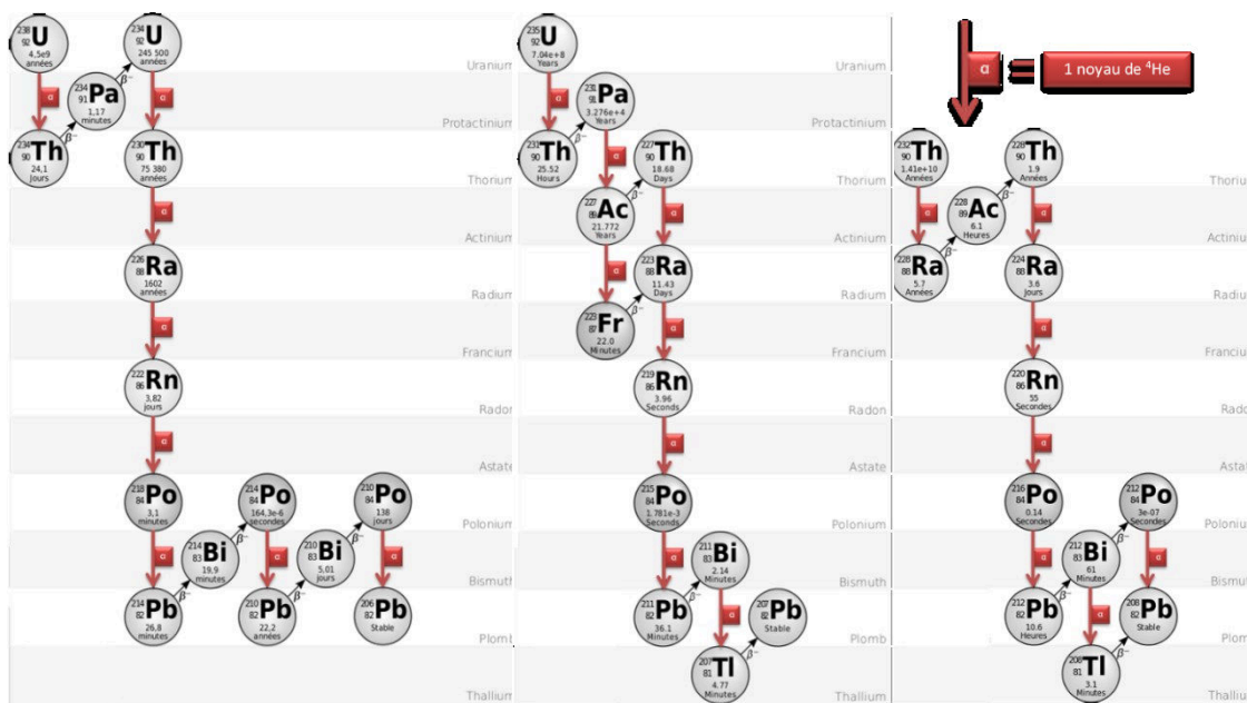
Figure 11 : Chaînes de désintégration de l' 238 U, de l' 235 U et du 232 Th et production d' 4 He associée, adapté de Wikipédia
