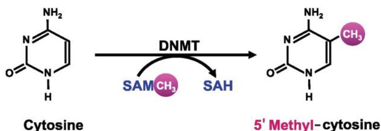
Figure 16. Représentation schématique de la méthylation de l'ADN, qui convertit une cytosine en 5' méthyl-cytosine, grâce à l'action méthyl-transferase (DNMT). SAM = S-adenosylméthionine; SAH = S-adenosylhomocystéine (Zakhari, 2013)
